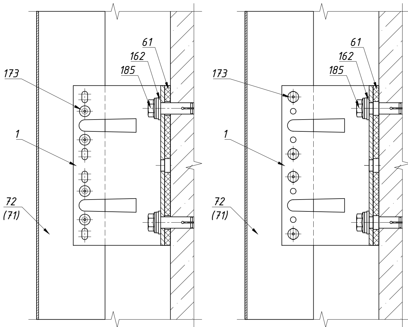
Фиксированная опора
