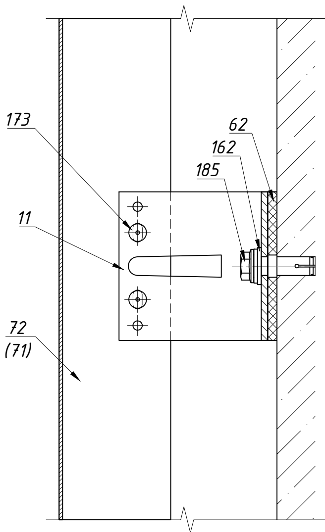
Подвижная опора
