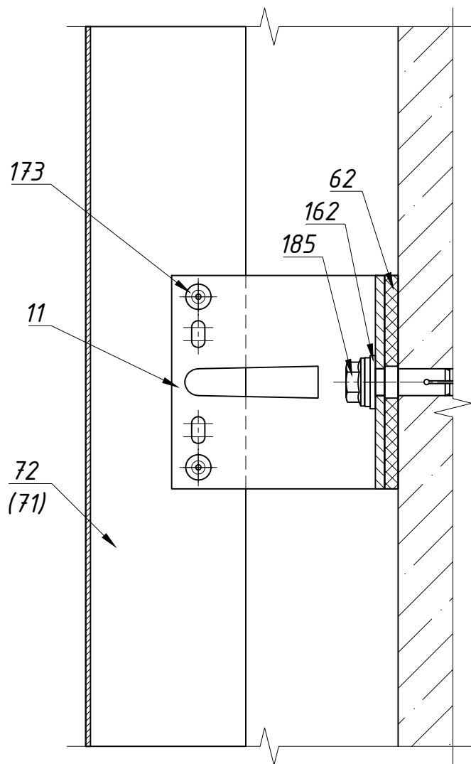
Фиксированная опора
